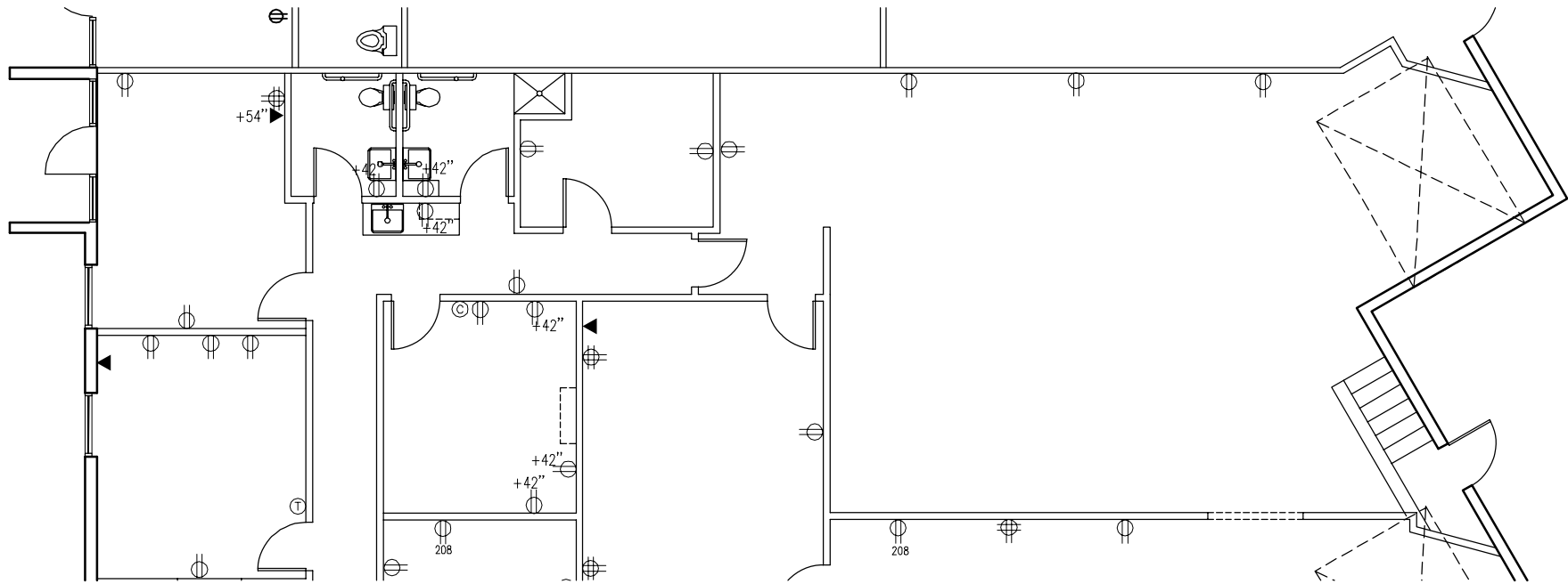
1 1 UNIT 103 SCALE: 3/32"=1'-0"
